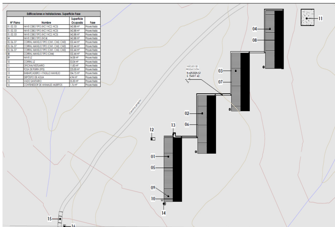
Fig. 2. Planta general de las instalaciones
